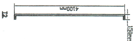
Ferro CA 50 Ø 16mm Comprimento total: 4400mm Quantidade: 30 peças
