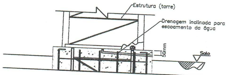
Posicionamento da drenagem
