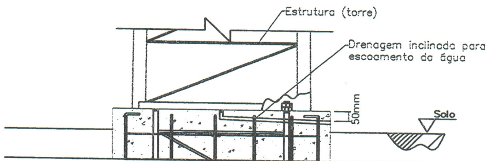
Posicionamento da drenagem
