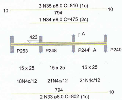
V21 ESC 1:50
