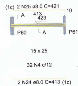
V10 ESC 1:50
