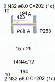
V20 ESC 1:50
