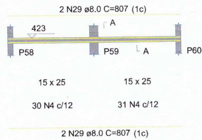
V9 ESC 1:50
