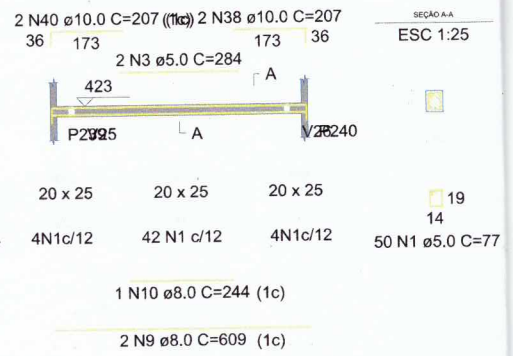
V2 ESC 1:50
