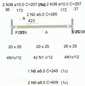
V1 ESC 1:50
