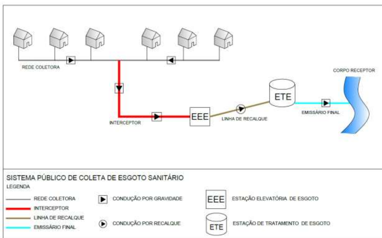
Figura 72: Croqui simplificado de um sistema de coleta de esgoto sanitário.
